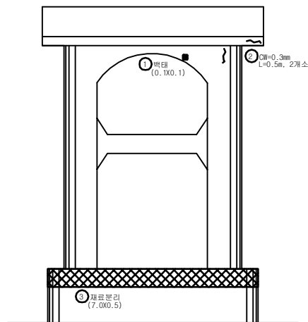
[ 정 면 ]
