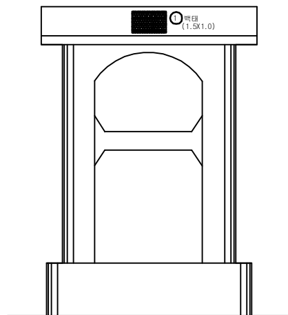
[ 정 면 ]
